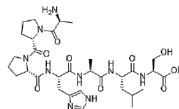
Ala-Pro-Pro-His-Ala-Leu-Ser
